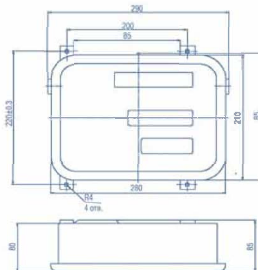
Габаритные размеры
